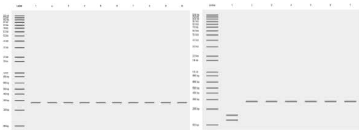
Gambar 2. Elektroforegram hasil restriksi dengan enzim Taq I secara in silico .
