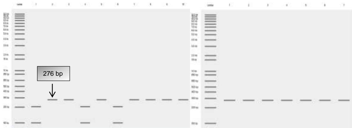
Gambar 1. Elektroforegram hasil restriksi dengan enzim Bgl II secara in silico .
